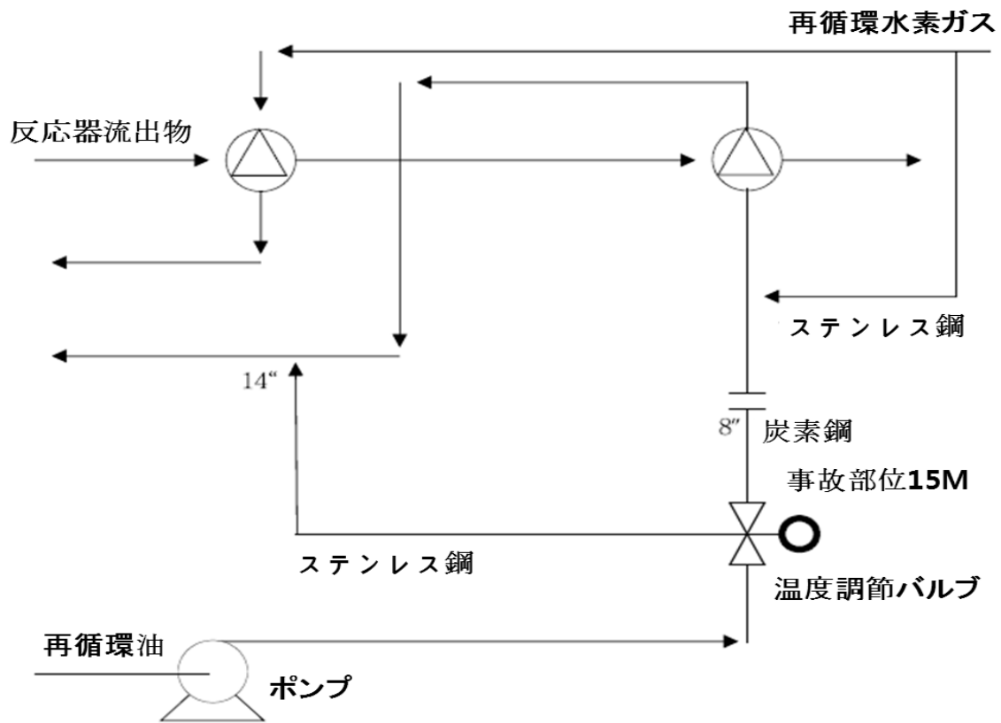
図。事故部位配管概路図
