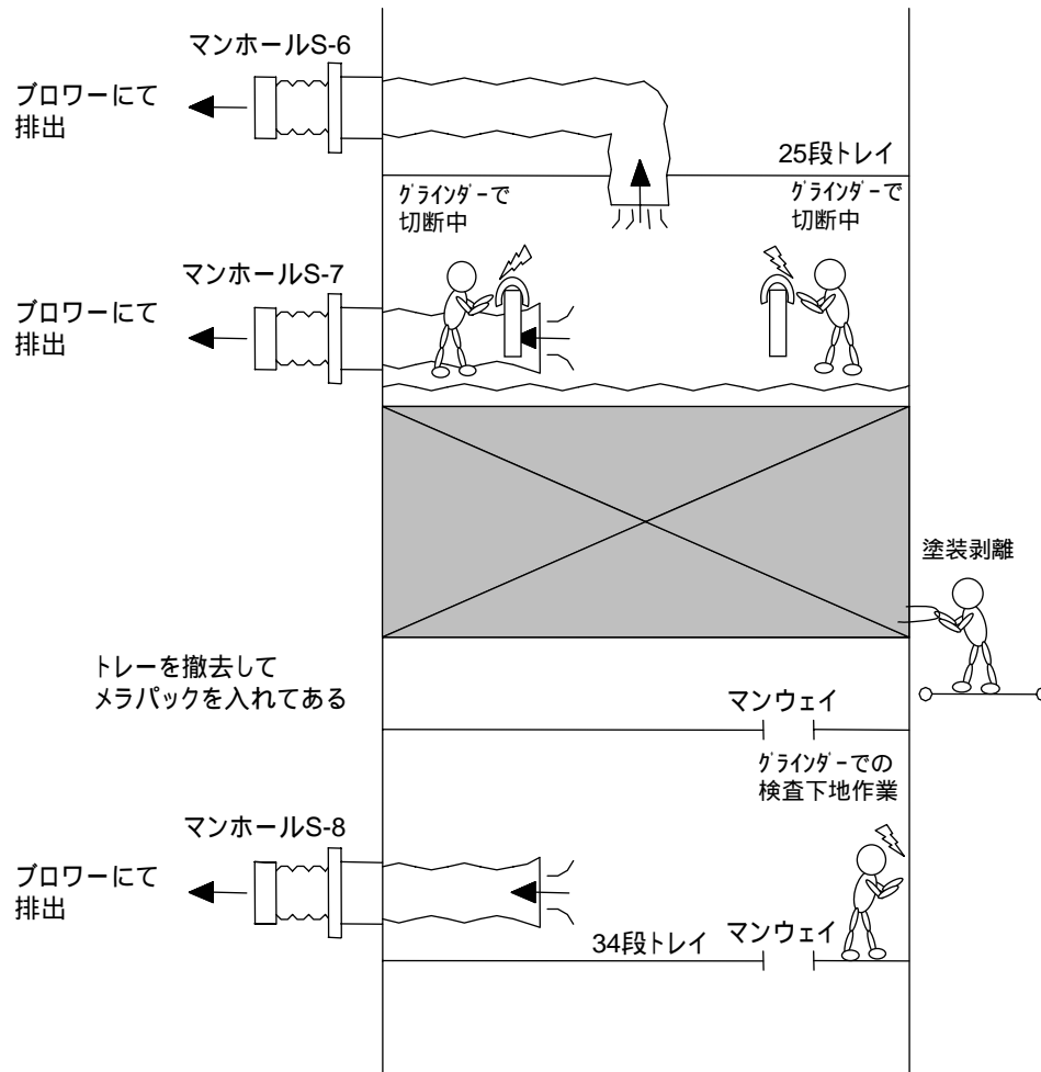
図 メラパック段の作業状況図
