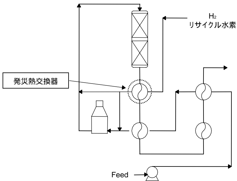
図 潤滑油水素化精製装置フロー図
