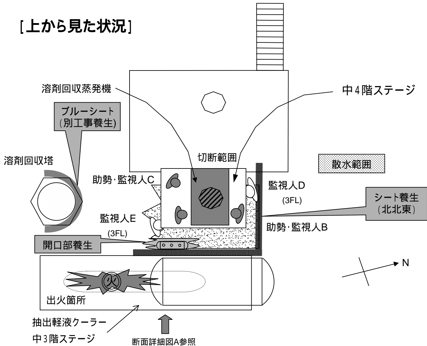
図1 要員配置と火気養生状況
