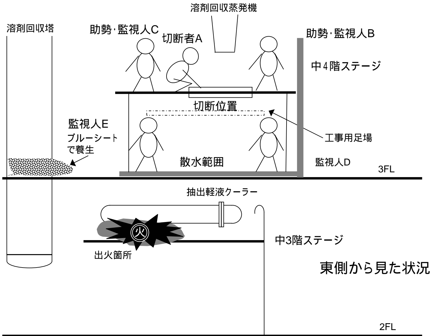
図2 切断作業詳細図(断面A)
