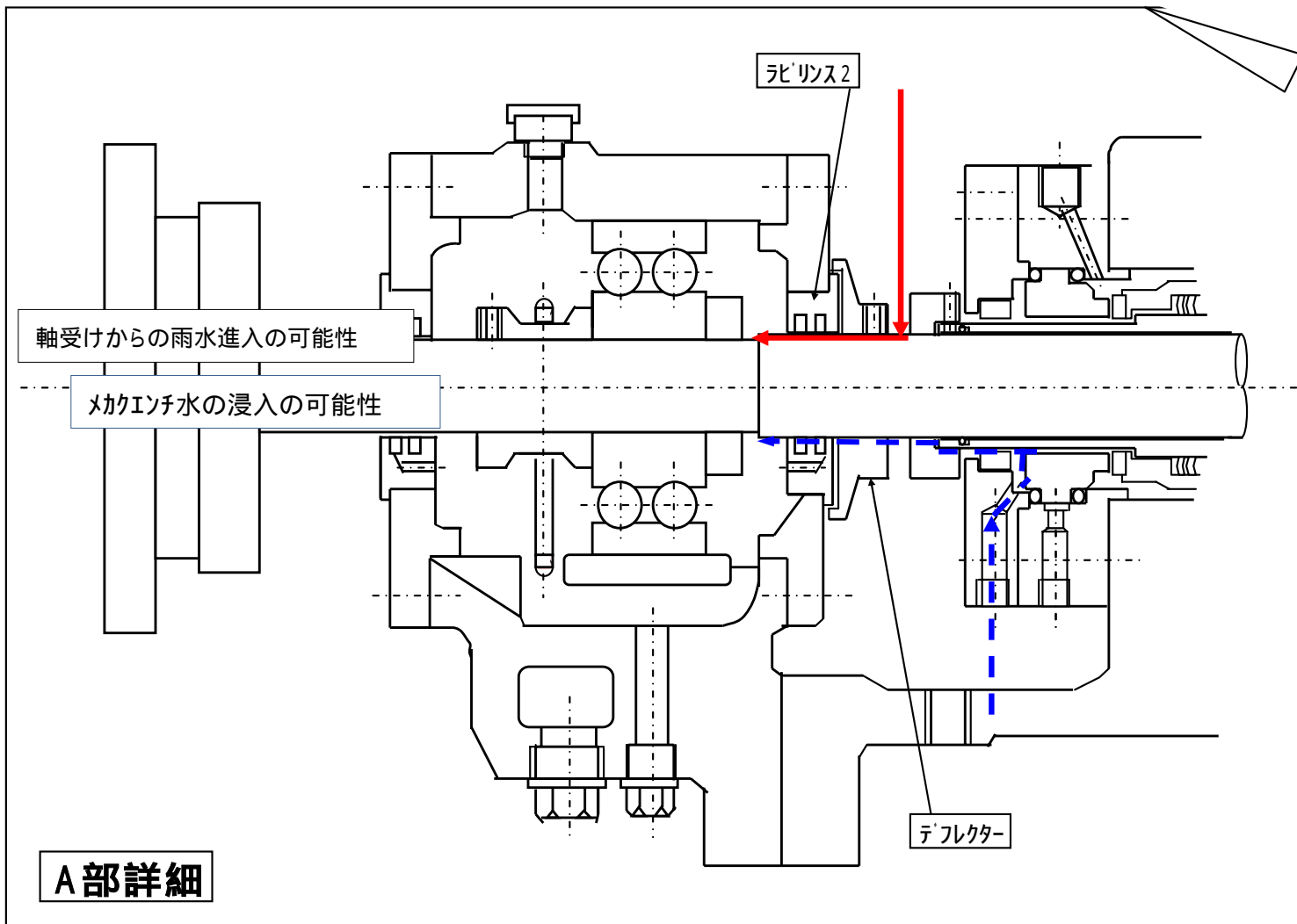
図2 A部詳細
