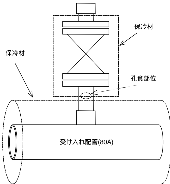
図 配管と保冷の概要
