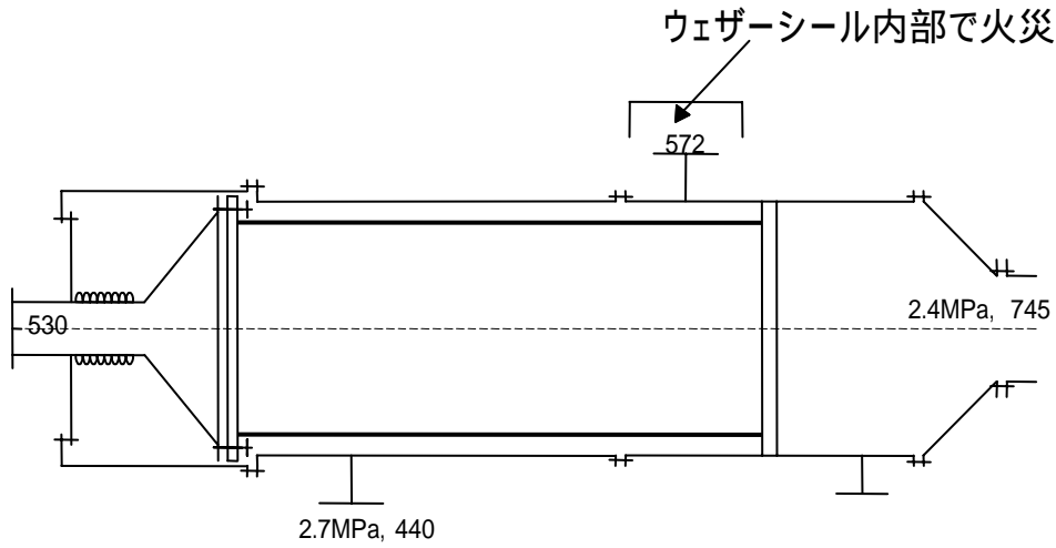
図1 熱交換器の概要
