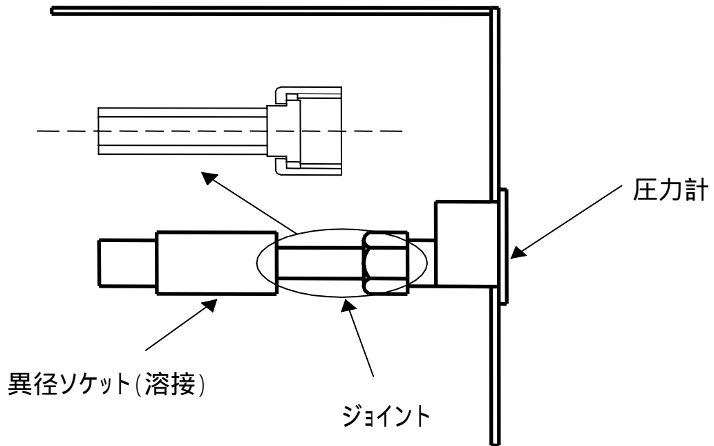
図 圧力計の取り付け概要
