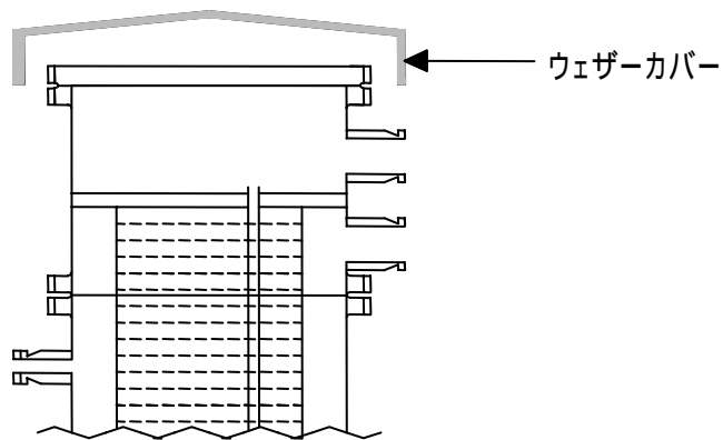
図1 縦型熱交換器のウェザーカバーの概要
