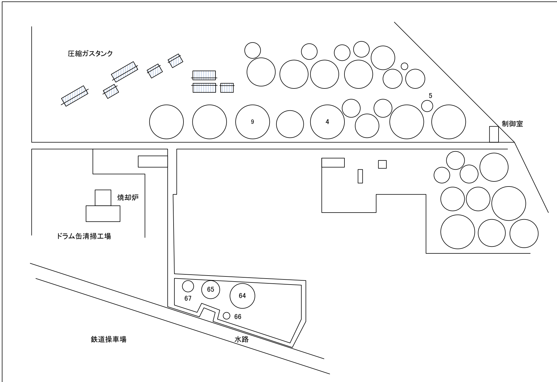
タンク配置図
