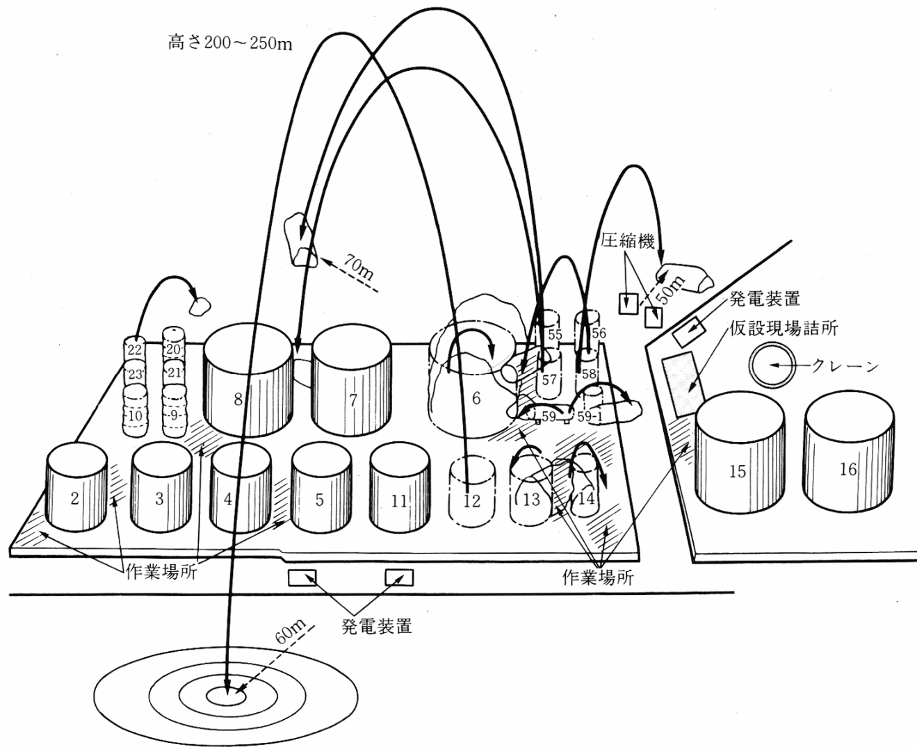
図 2 作業場所等の配置状況とタンク爆発状況
