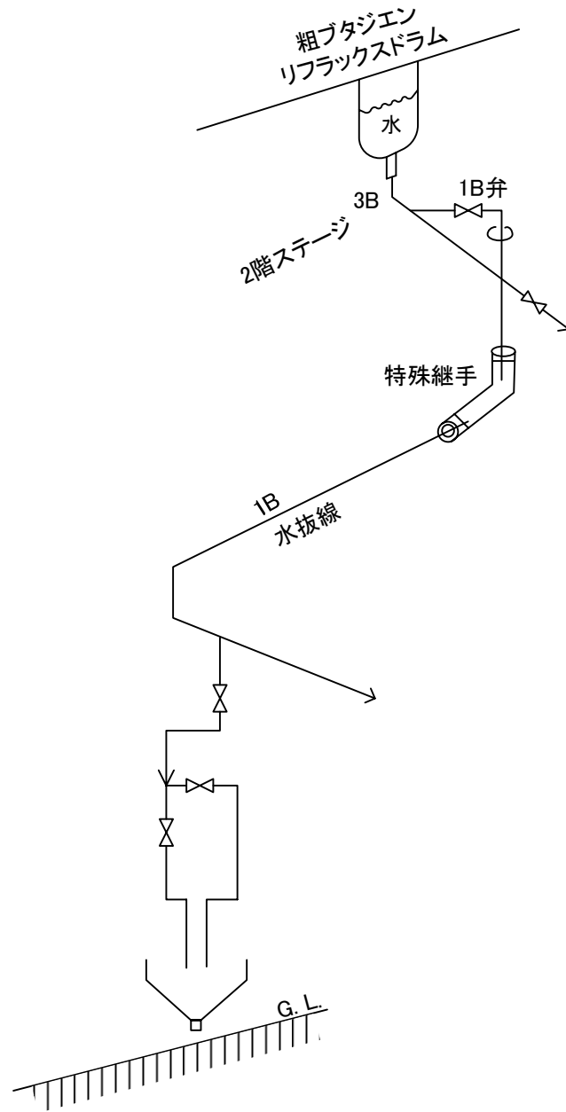
図3 水抜線図
