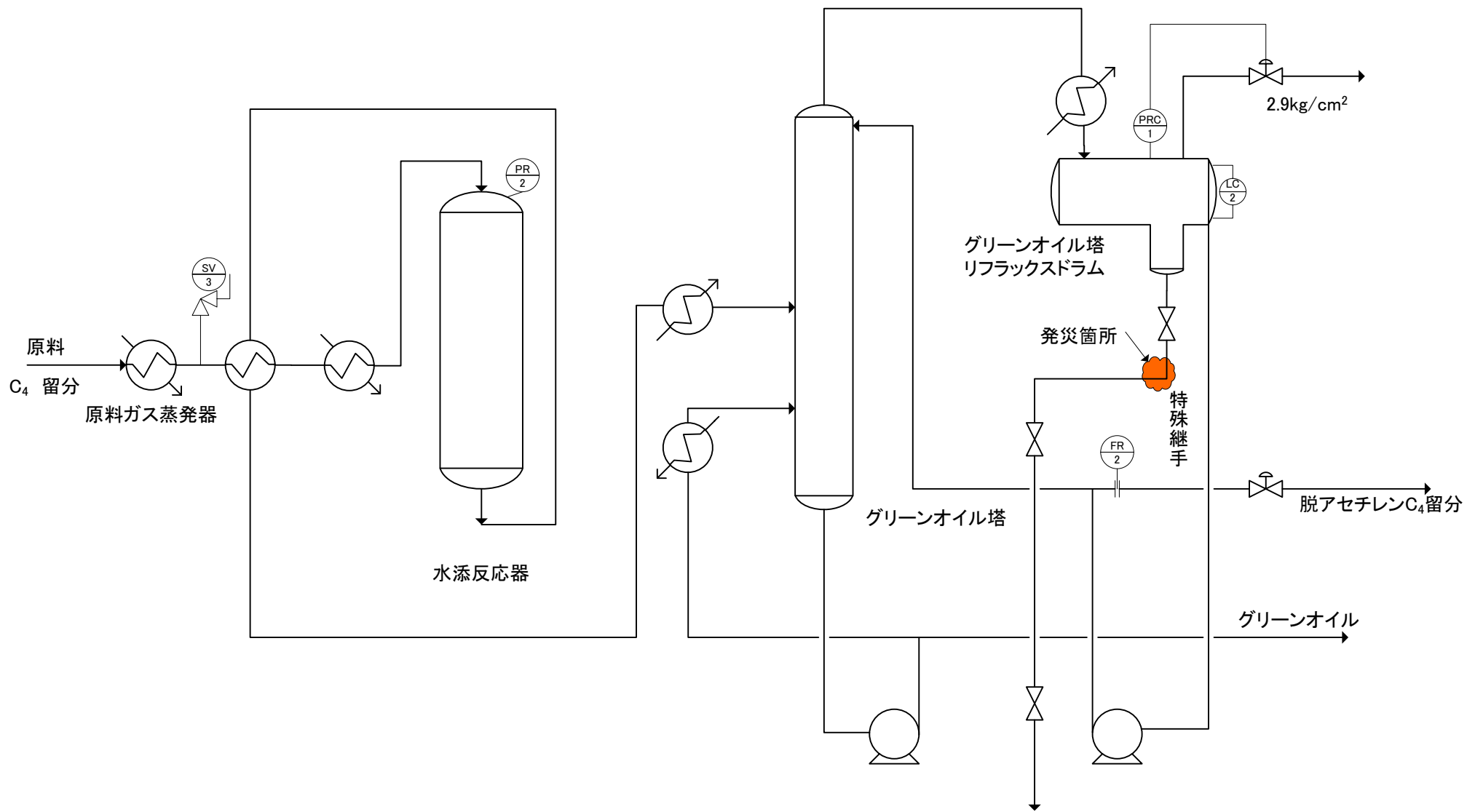
図1 ブタジエン製造装置前処理部門系統図
