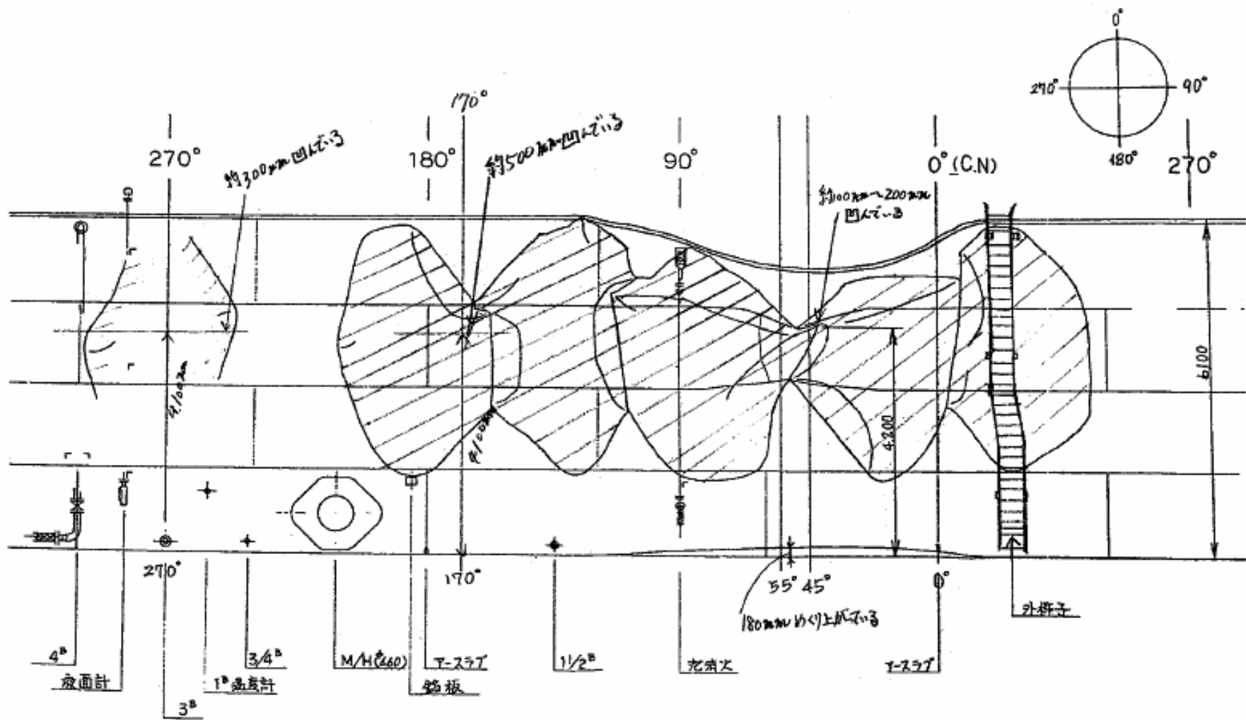
側板変形状況展開図
