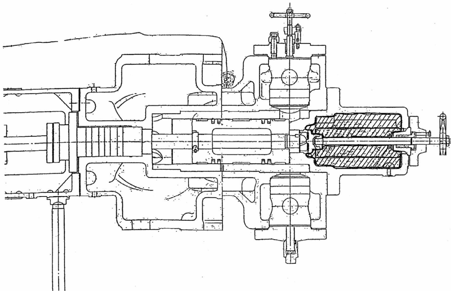
クリアランスポケットバルブ
