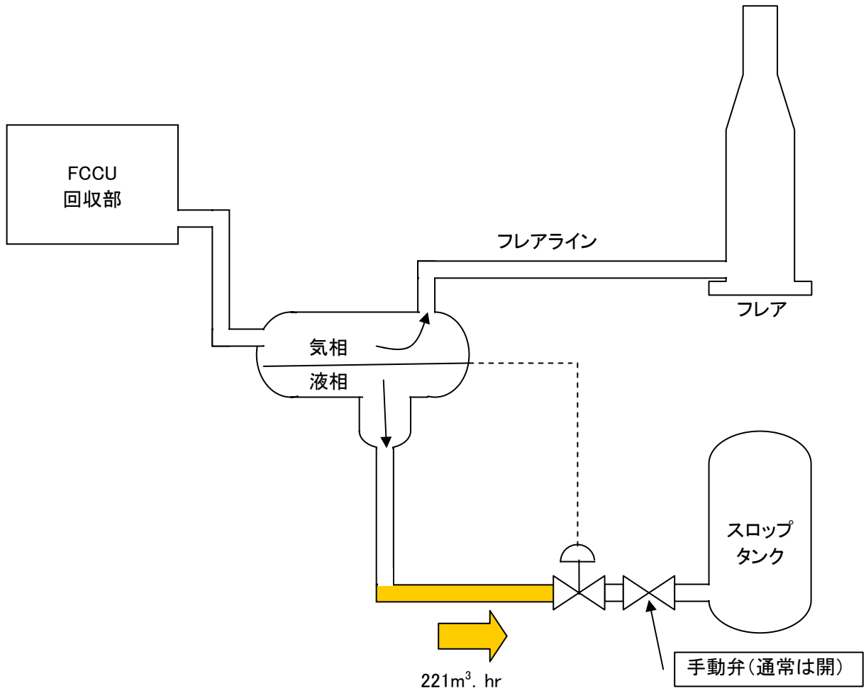
図 2 フレアノックアウトドラムまわり(変更前)
