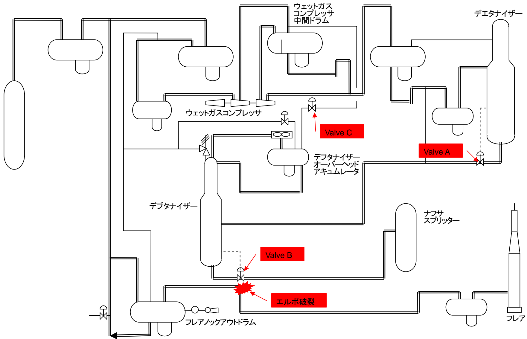
図1 プロセスフロー図
