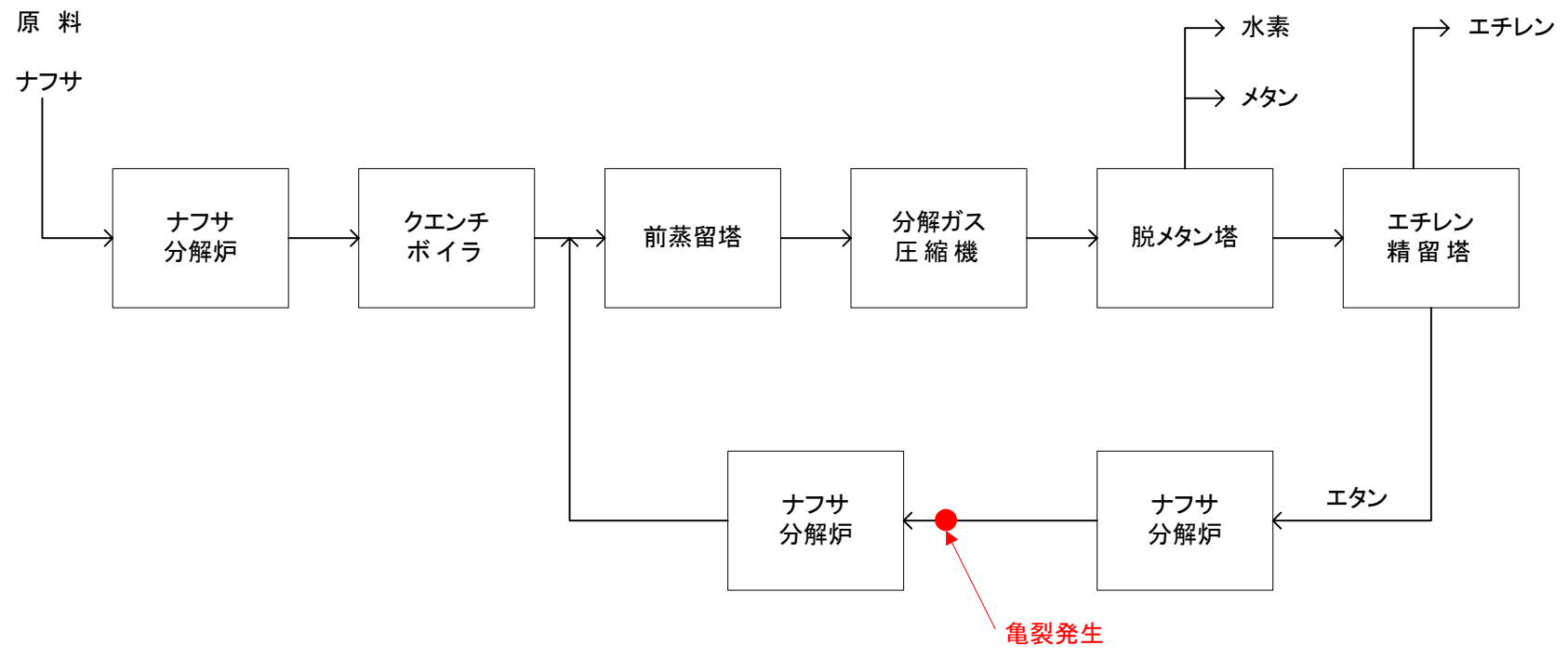
図1 プロセスのブロック線図
