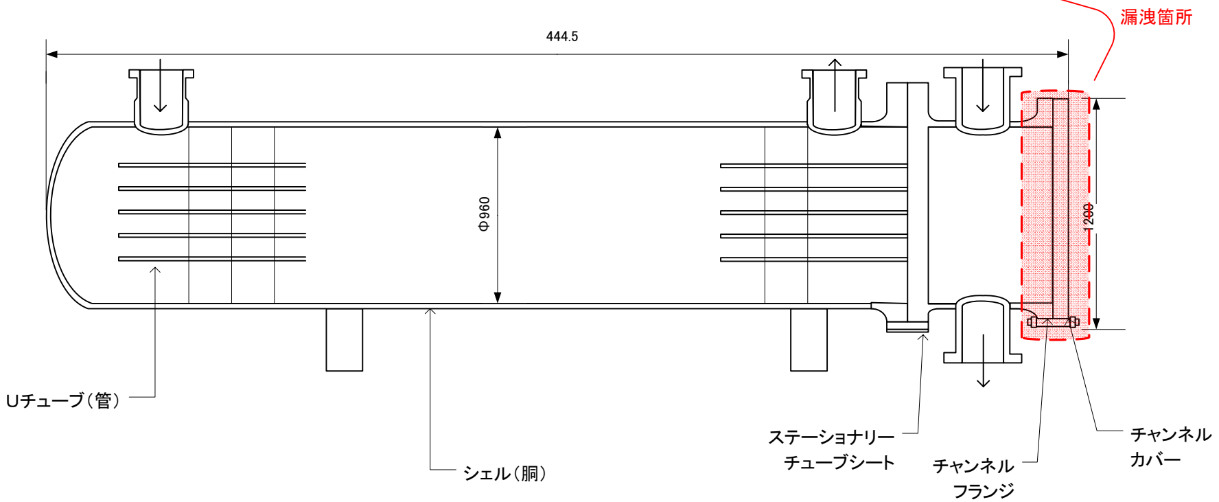
図2 熱交換器
