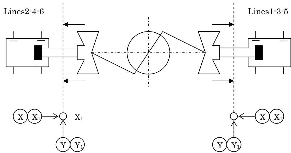
図3 往復動式コンプレッサの配置図
