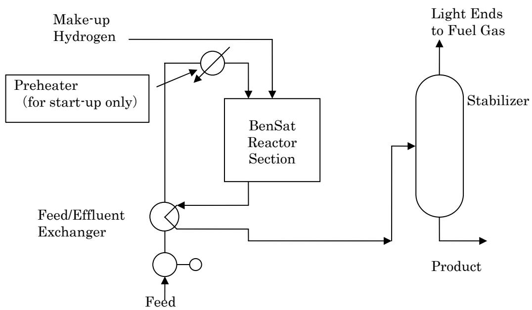
図 2 BenSat 廻りのプロセスフロー概略図
