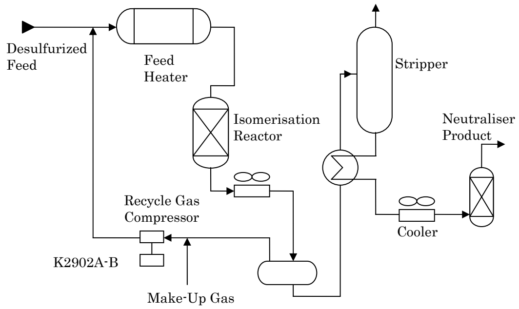
図1 プロセスフロー概略図
