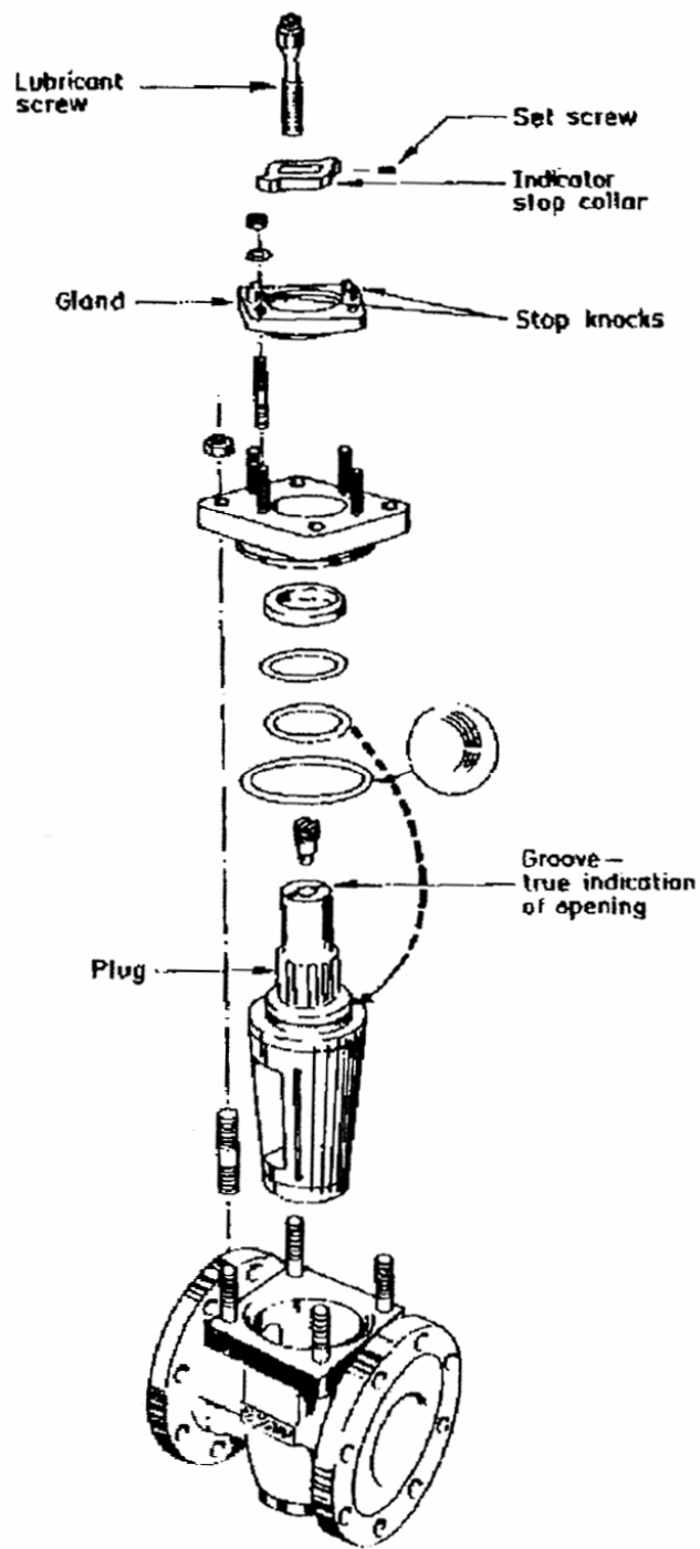
図1 プラグバルブ概略図
