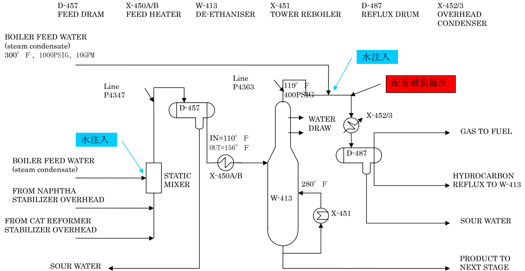
図 1 飽和ガスプラントプロセスフロー図
