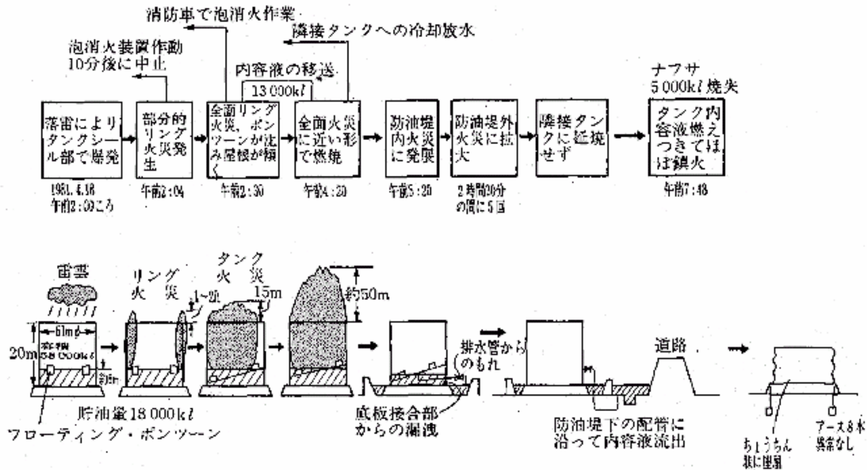
図3 タンク火災・出火から鎮火までの推移
