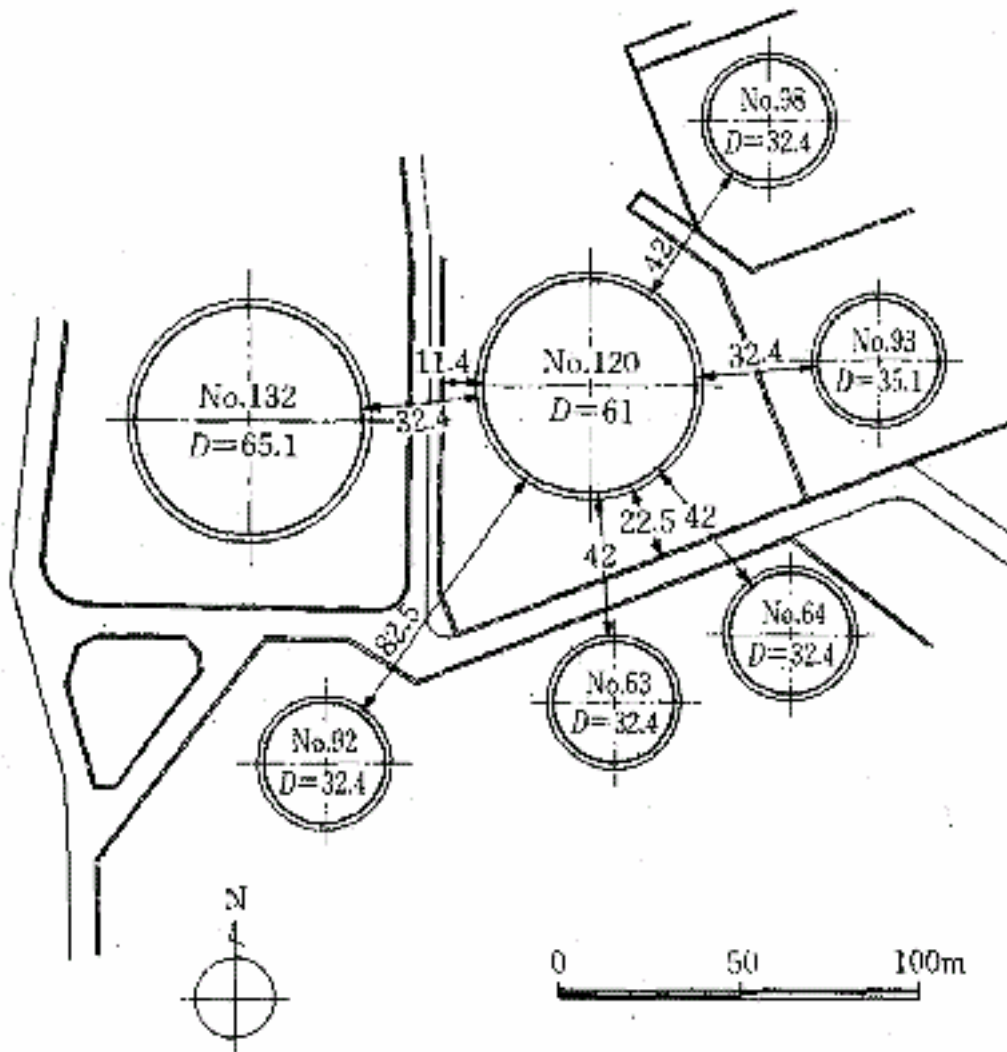
図 2 タンク配置図
