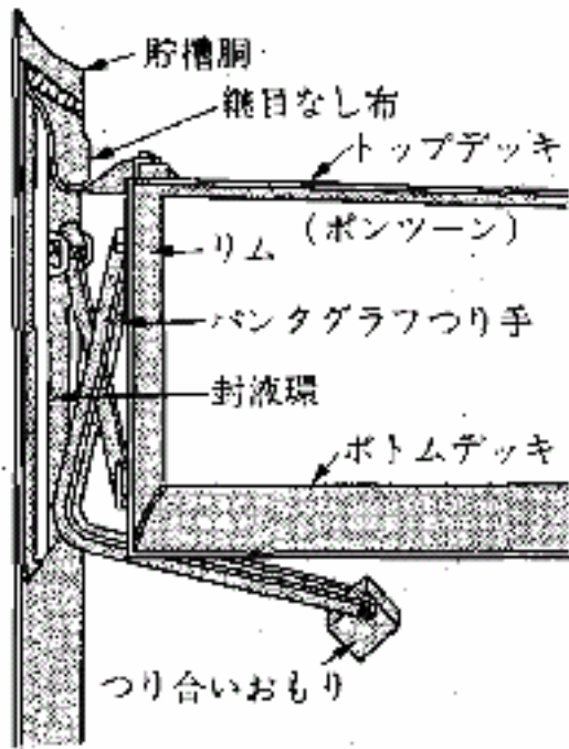
図1 シングルデッキ推定図
