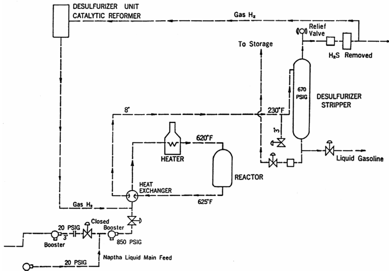
図 ガソリン改質装置概略フロー
