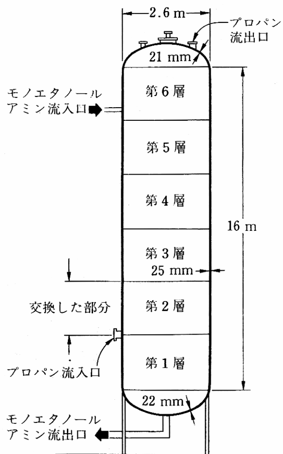
図1 圧力容器の構成
