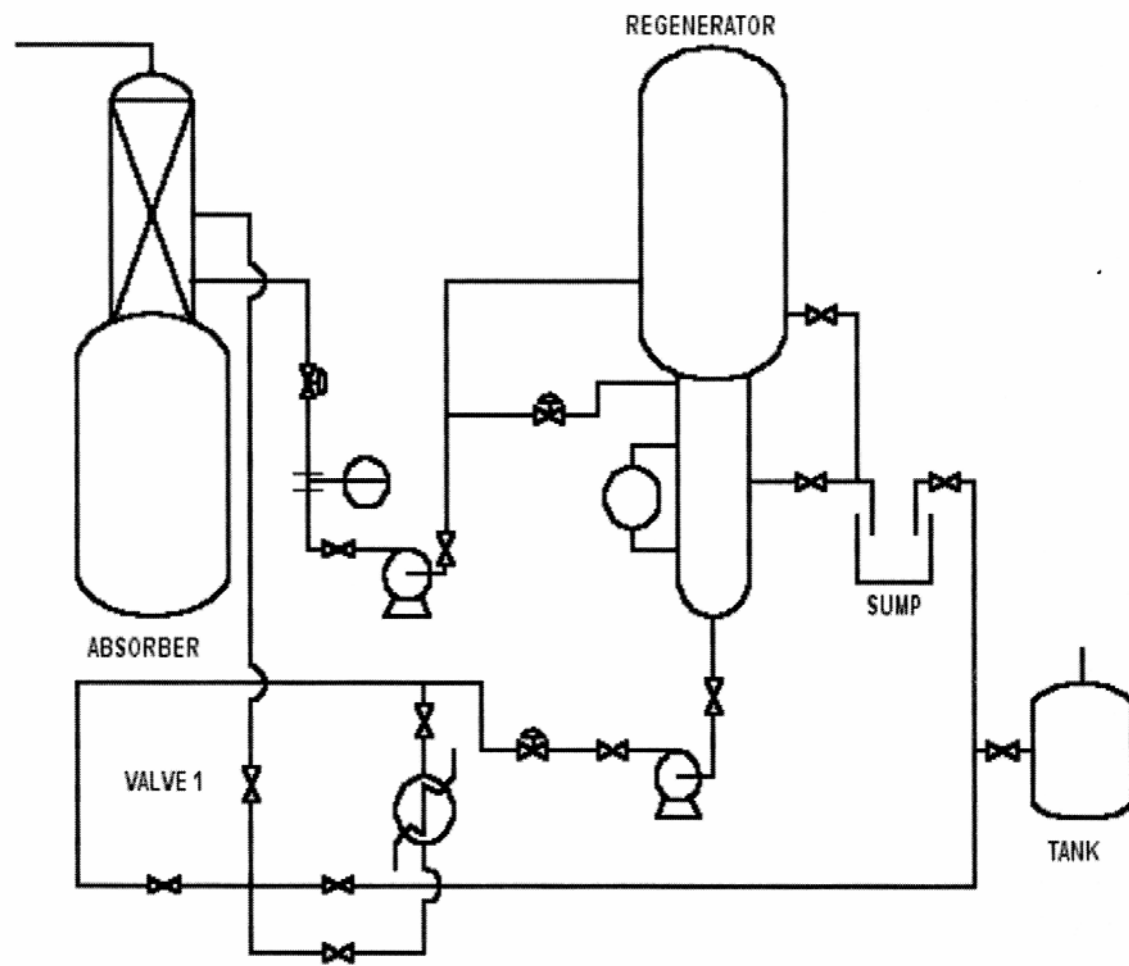
図 二酸化炭素除去システムプロセスフロー
