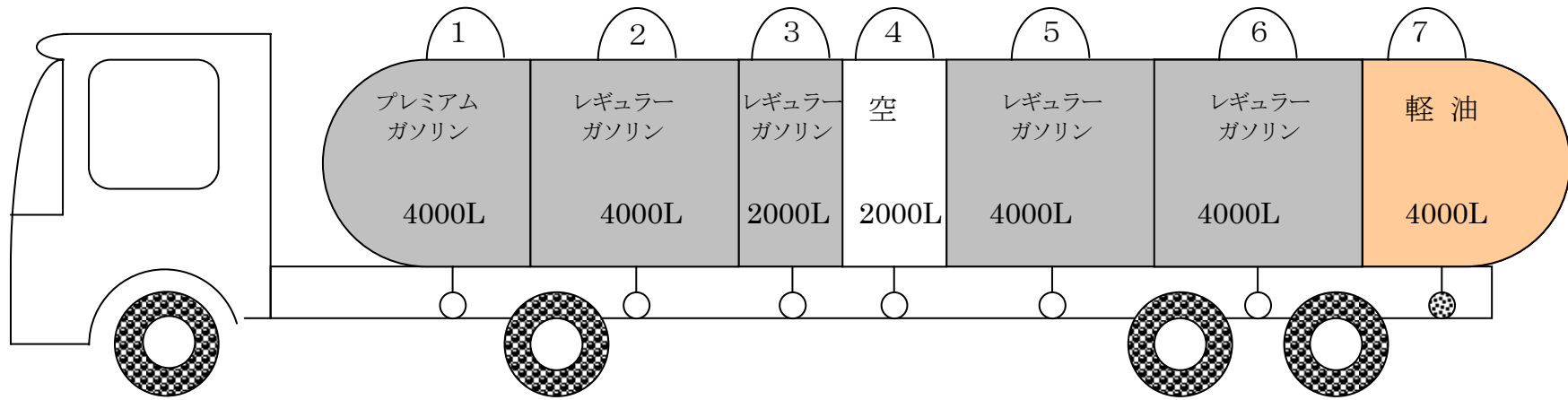
図1 ローリーハッチ割付け図
