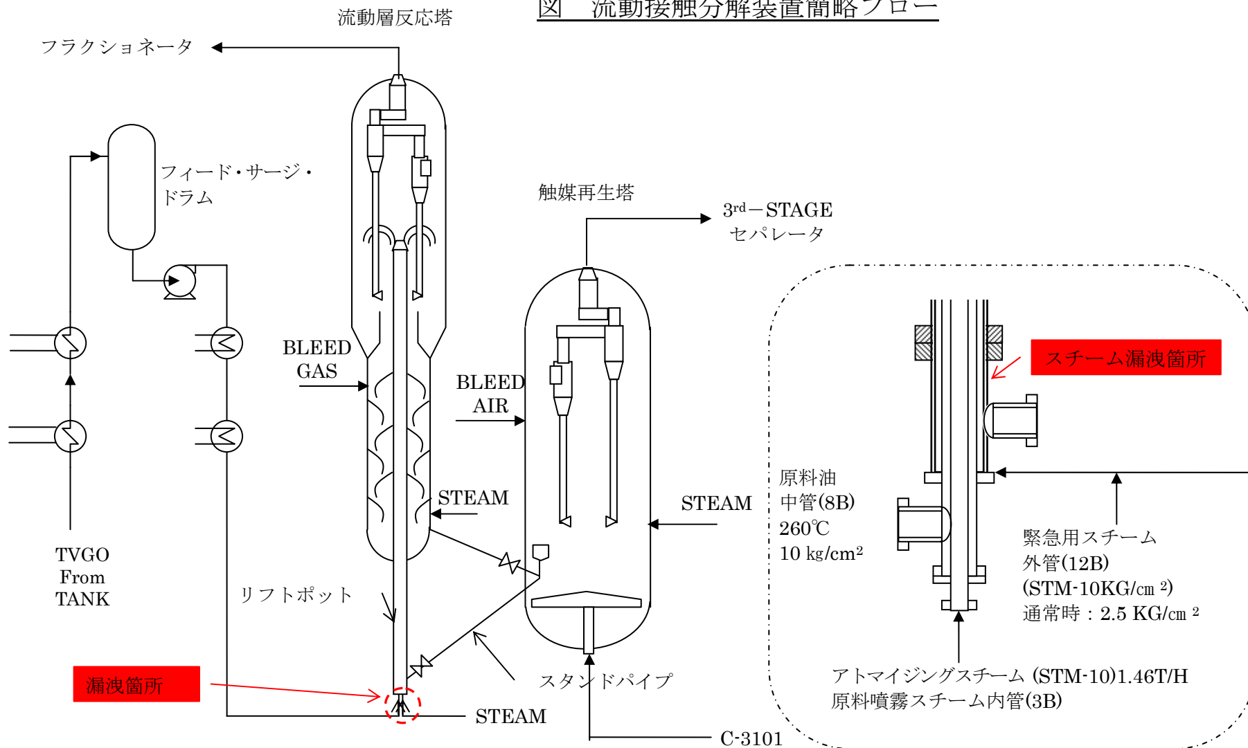
図 流動接触分解装置簡略フロー
