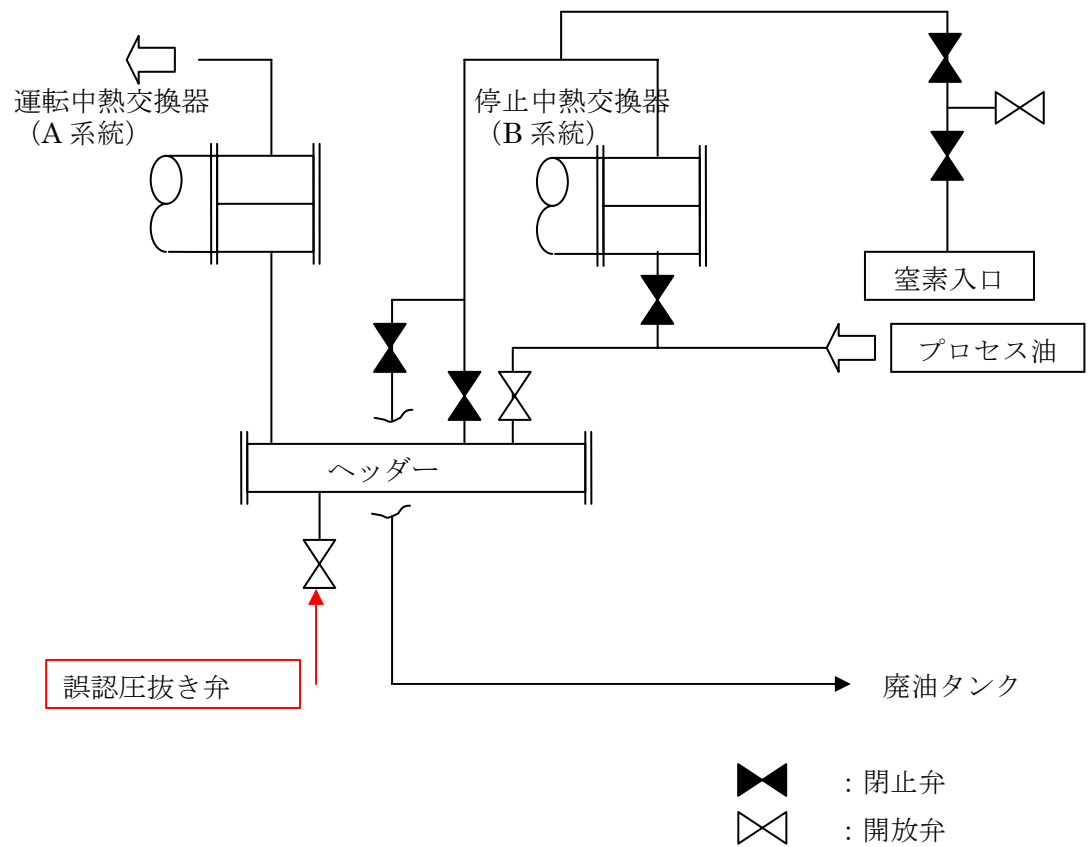
図 熱交換器付近配管略図
