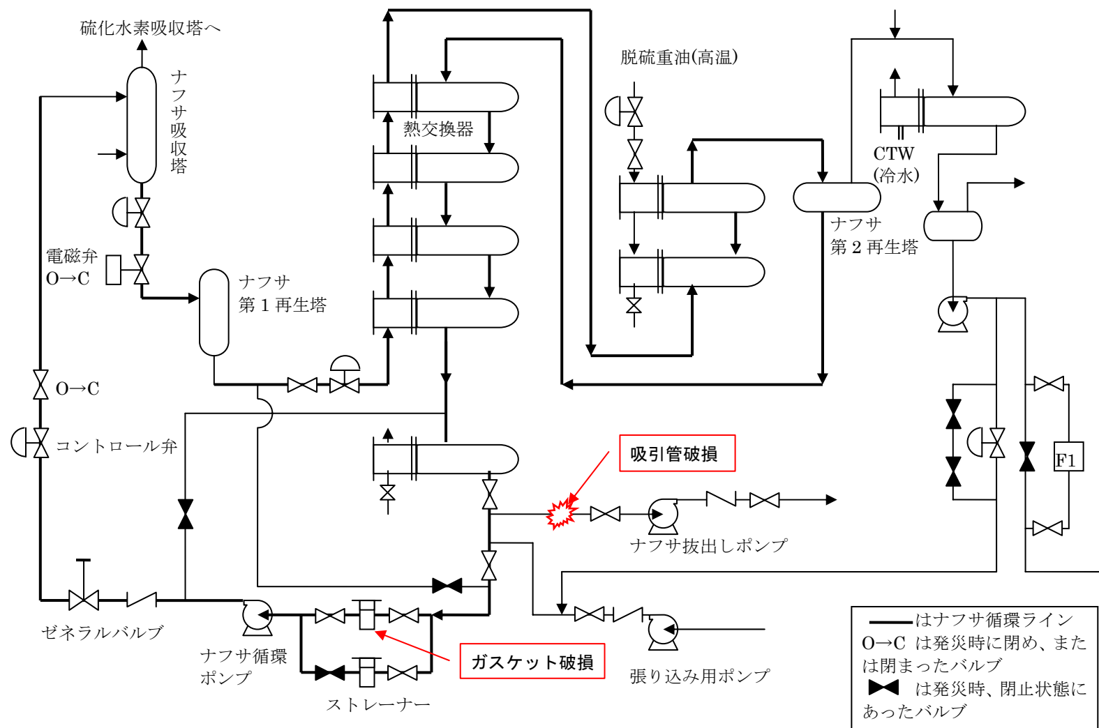
図 ナフサ循環系フローと弁開閉状況
