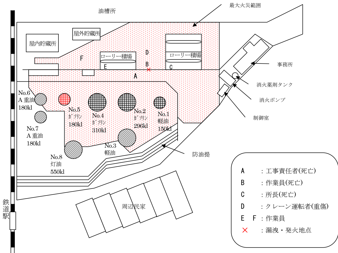
図 油槽所配置及び人員配置(推定含む)
