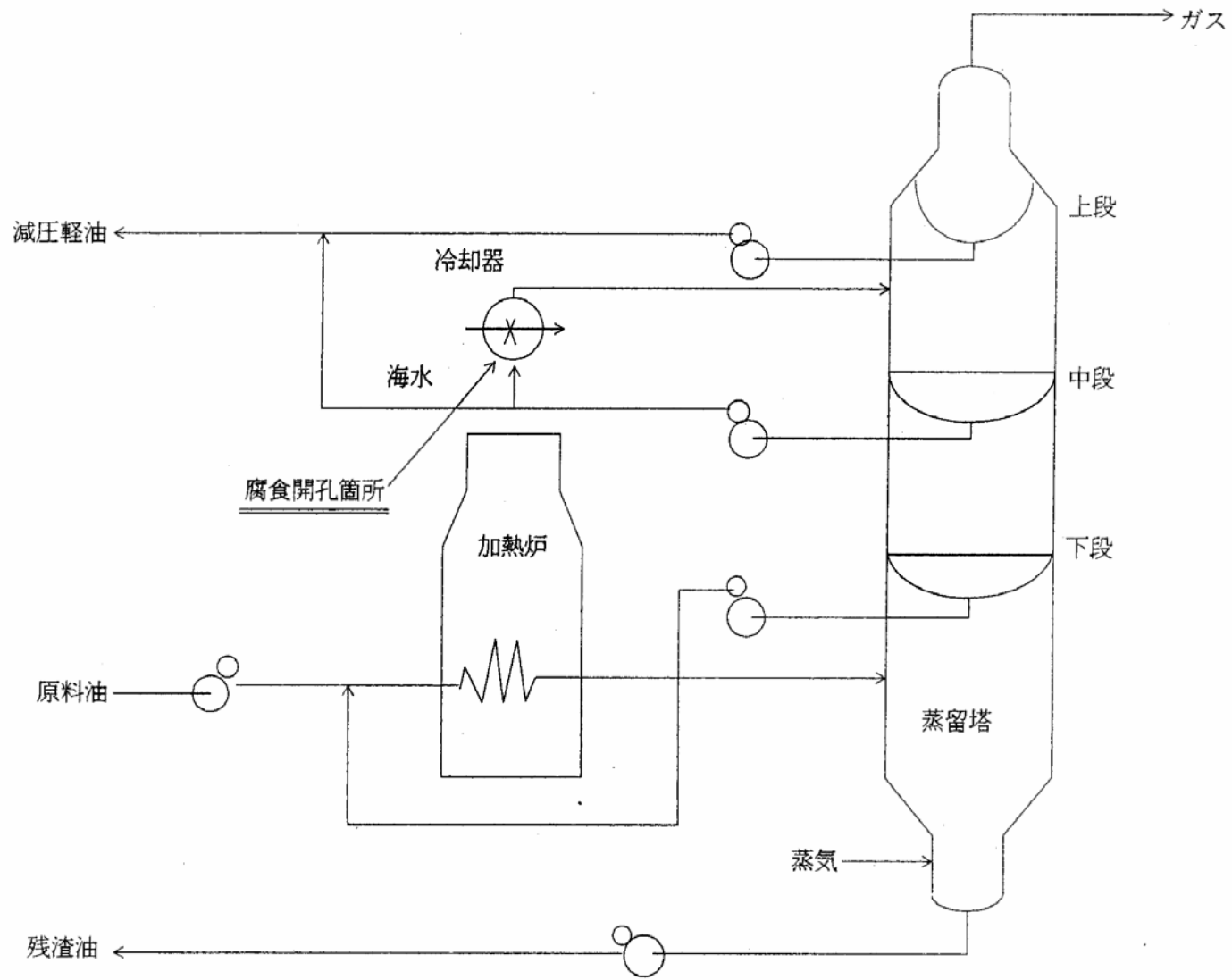
図 減圧蒸留装置工程略図
