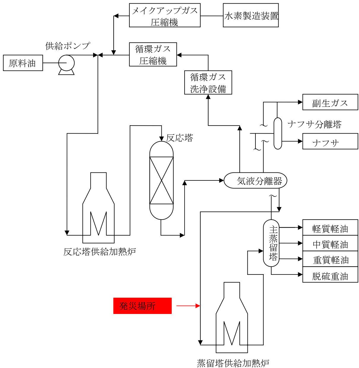
図 重油直接脱硫装置概略フロー
