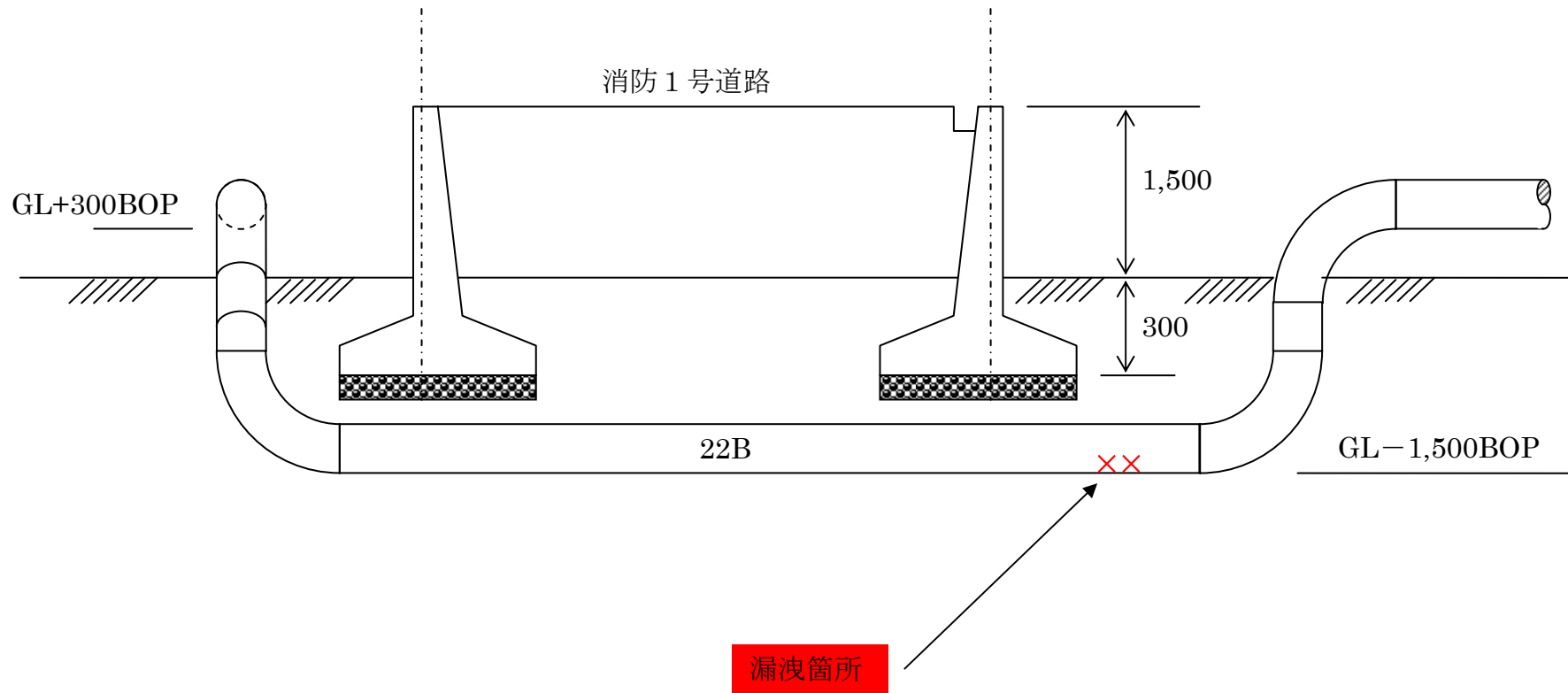
図 埋設配管漏洩箇所
