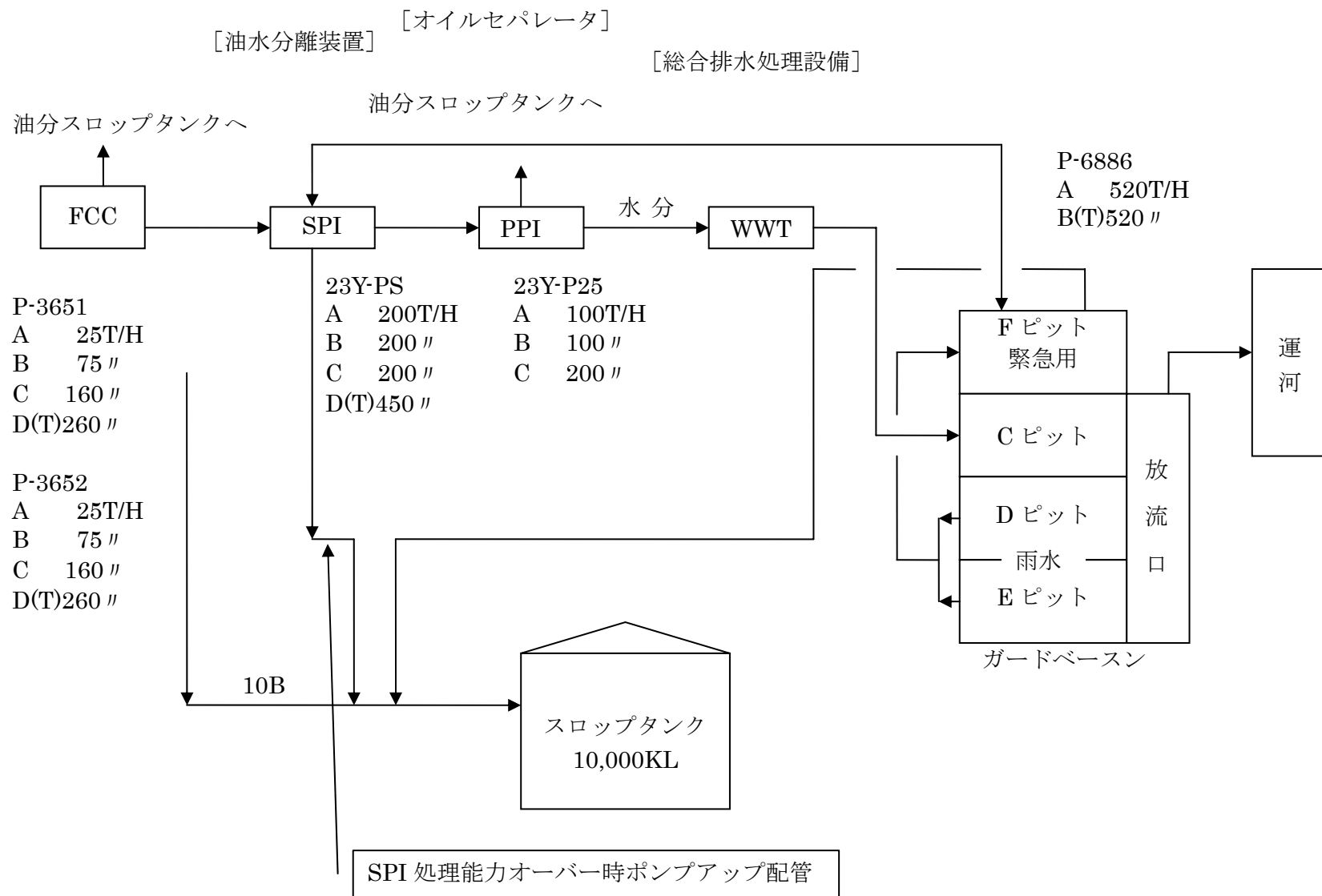
図2 含油排水フロー図
