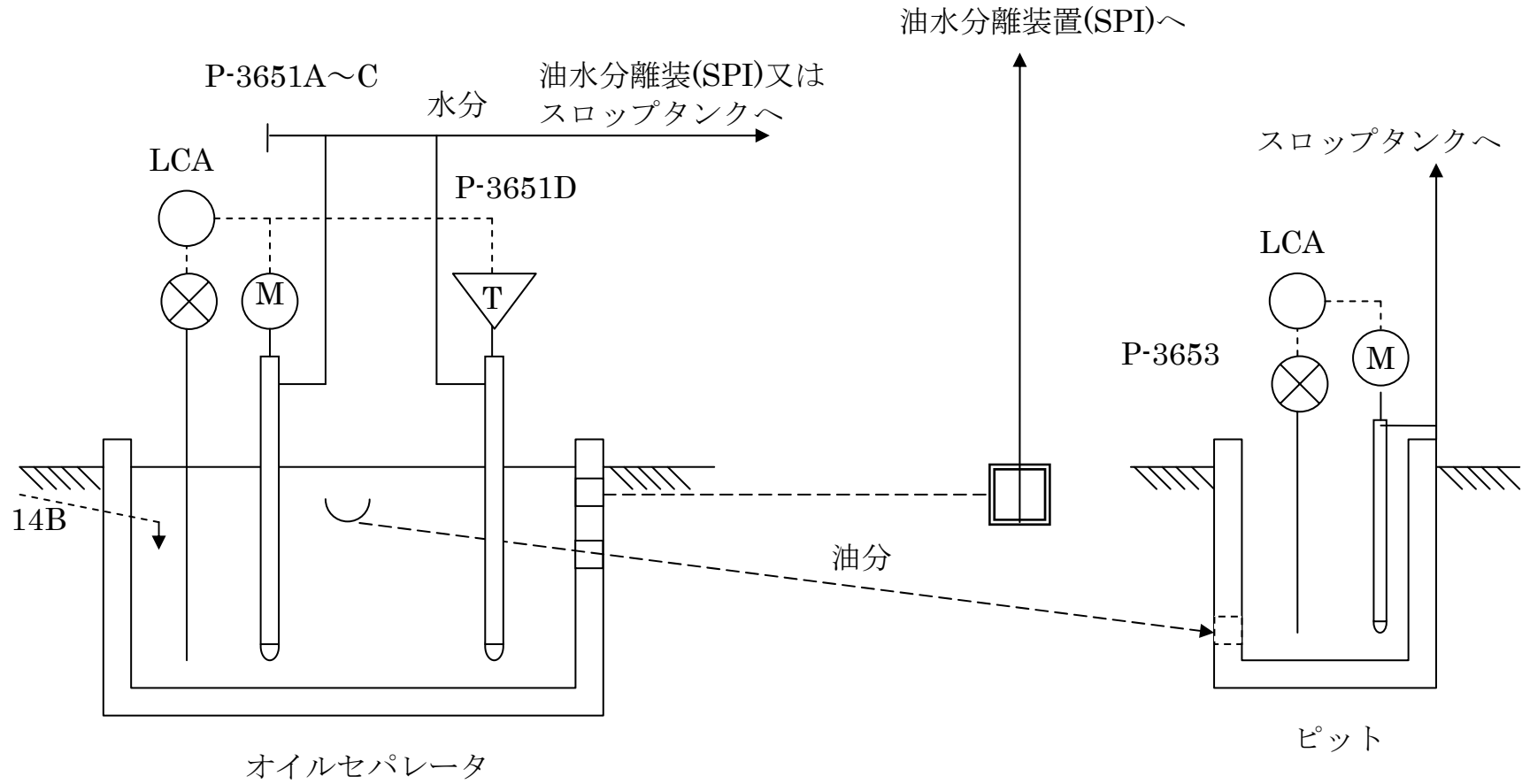
図1 流動接触分解装置含油排水フロー図
