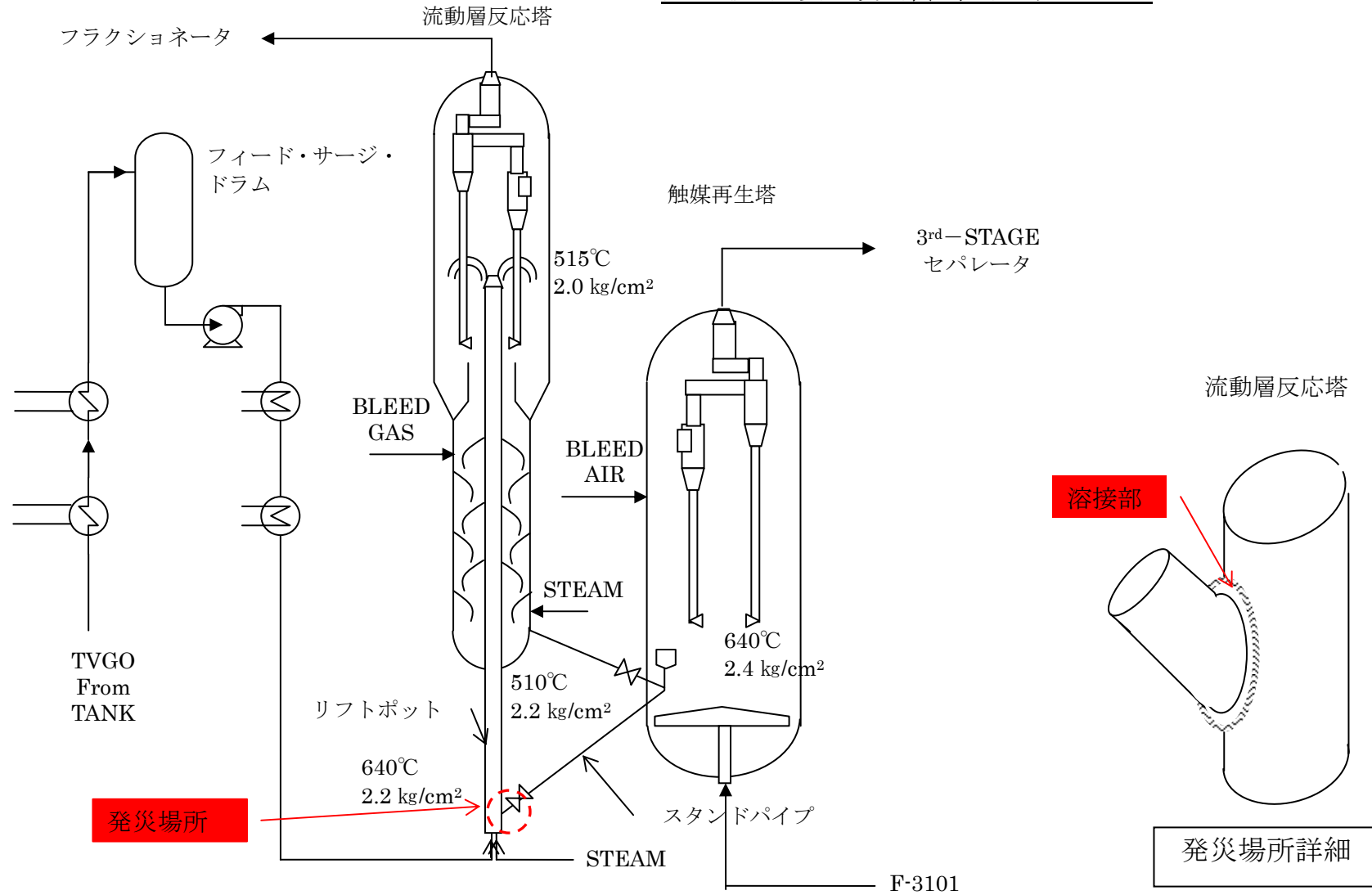
図 流動接触分解装置簡略フロー
