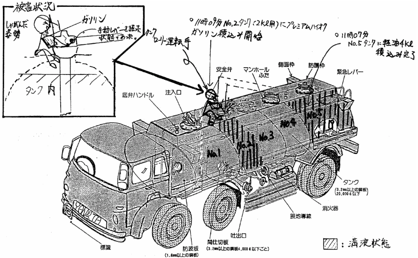
図1 タンクローリー運転手積込状況図
