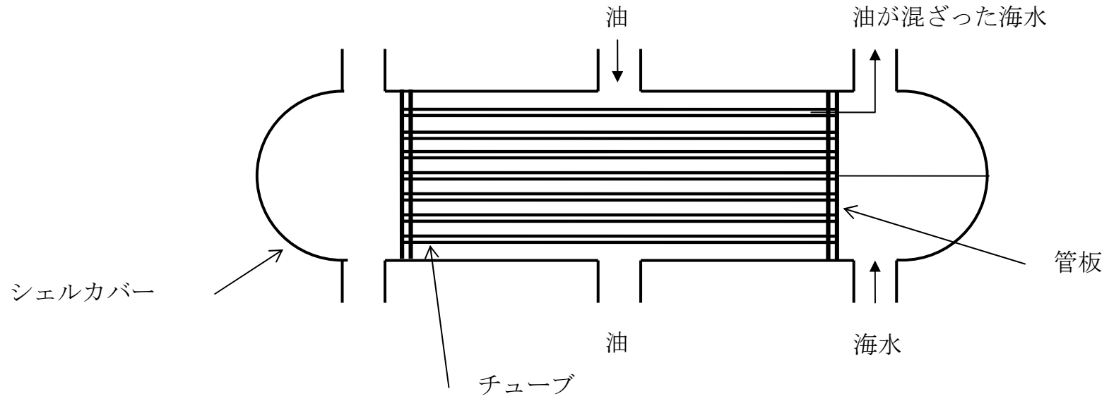
図2 潤滑油冷却器
