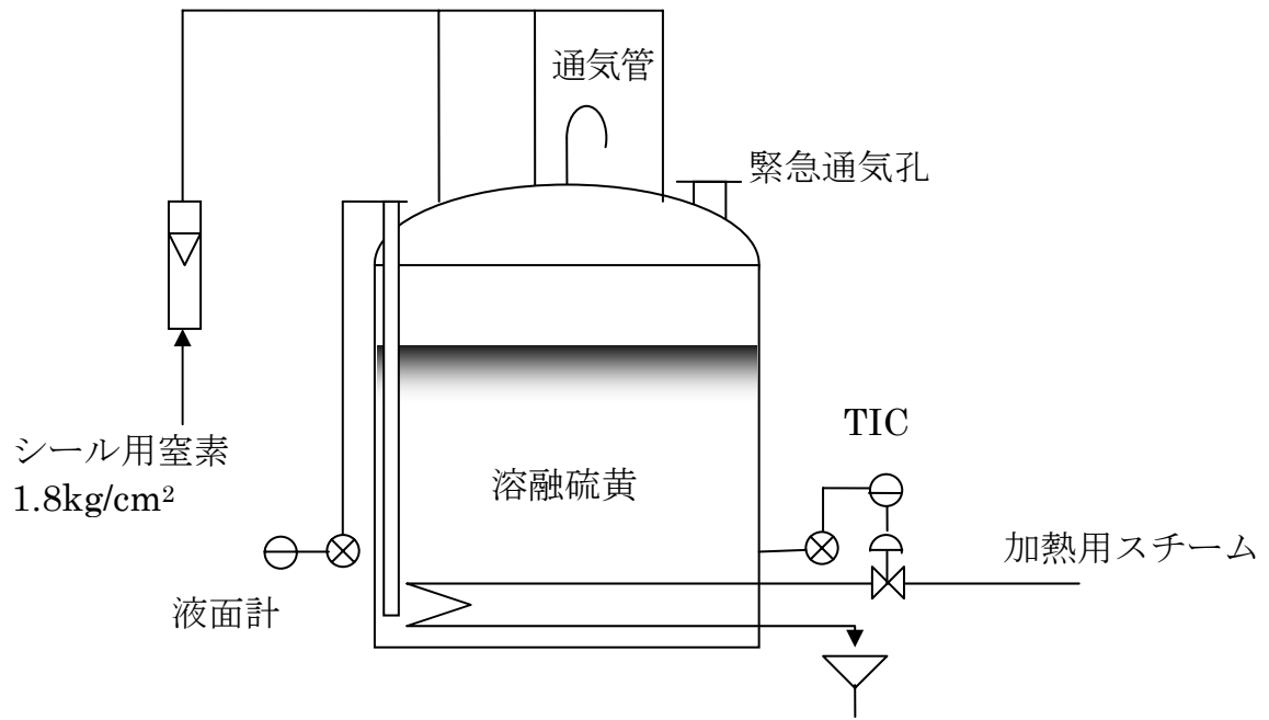
図 溶融硫黄タンクシステム
