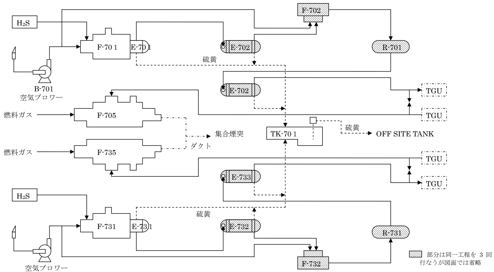
図 硫黄回収装置概略フロー
