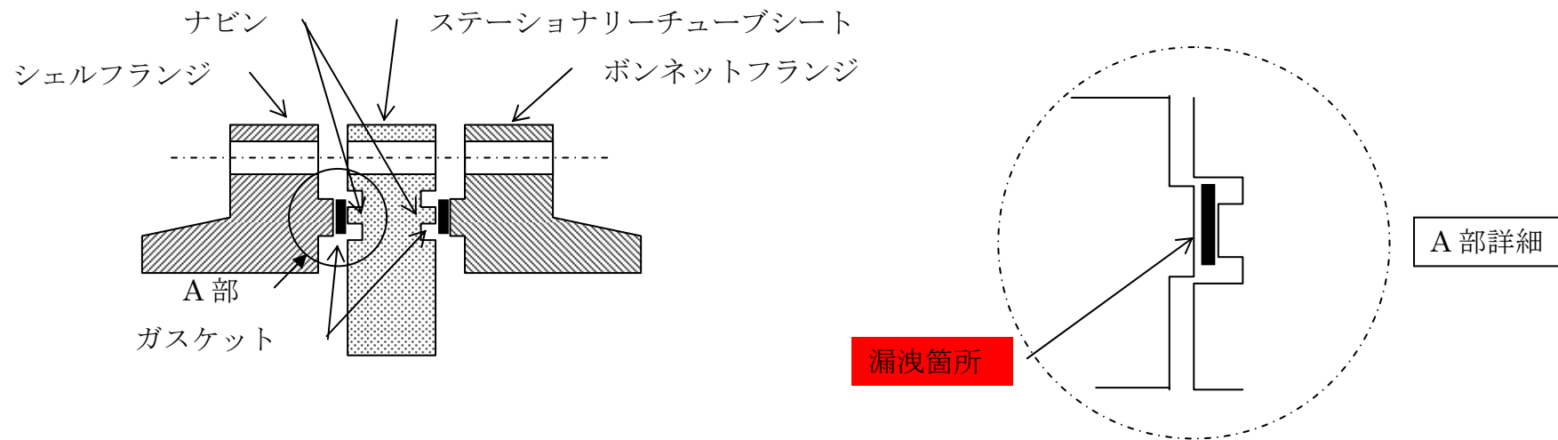
図3 熱交換器詳細
