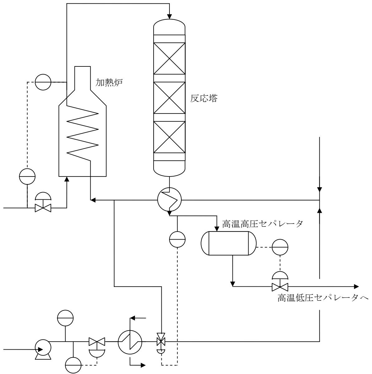
図 灯軽油水素化脱硫装置簡略フロー
