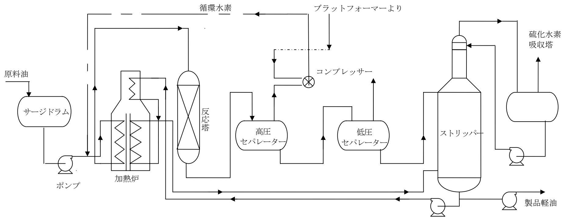
図 軽油水素化脱硫装置フロー
