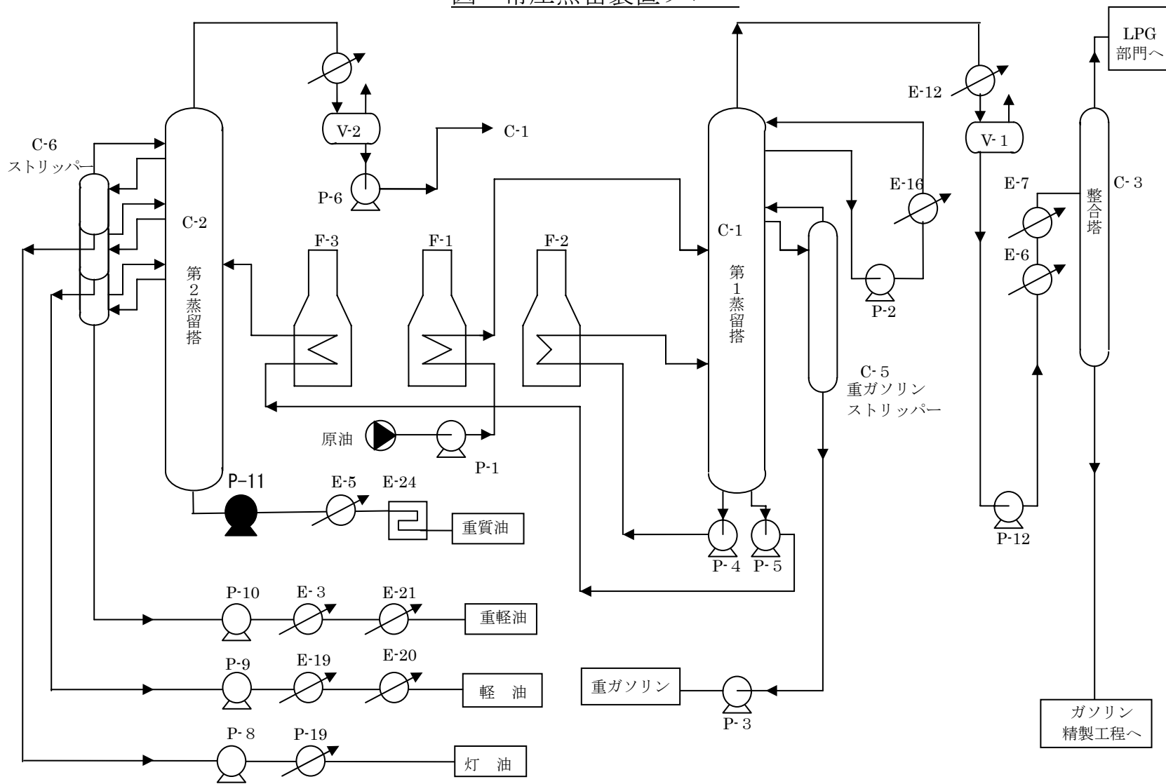
図 常圧蒸留装置フロー
