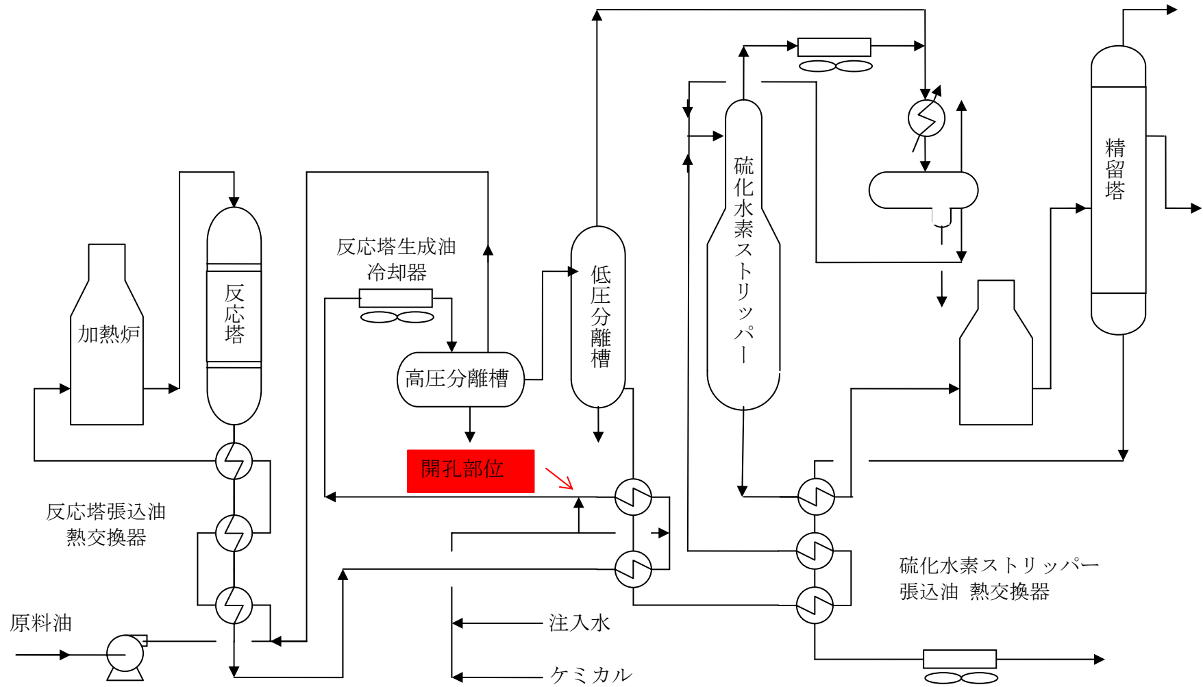
図1 アイソマックス装置概略フロー
